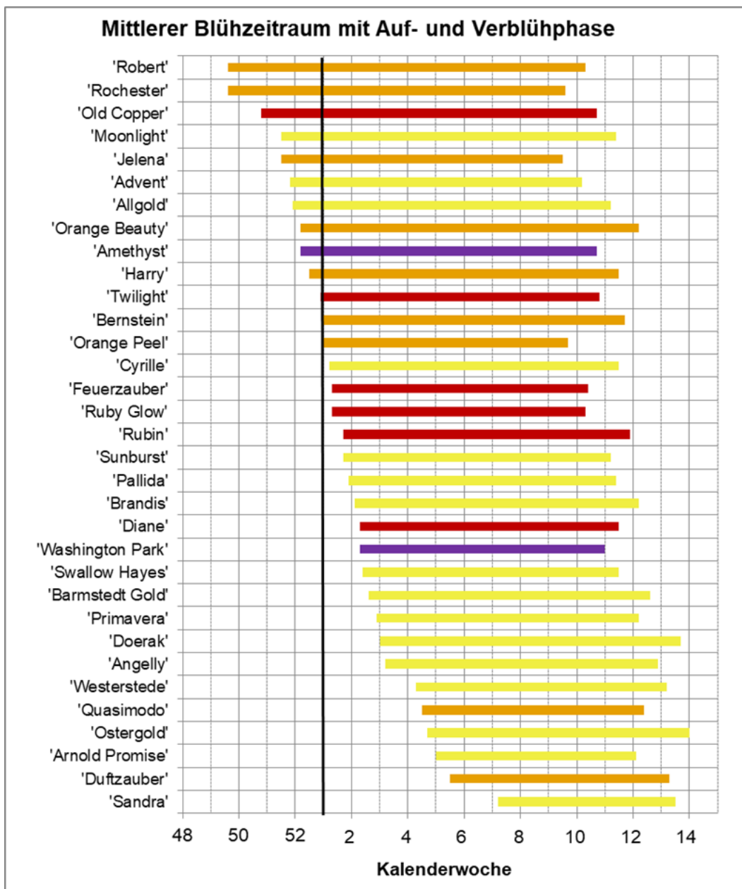
Abb. 3: Blühzeitenkalender (inklusive Auf- und Verblühphase) der geprüften Zaubernuss-Sorten im Mittel über alle Sichtungstandorte. Die Balkenfarbe zeigt den Hauptfarbton der Blüten
